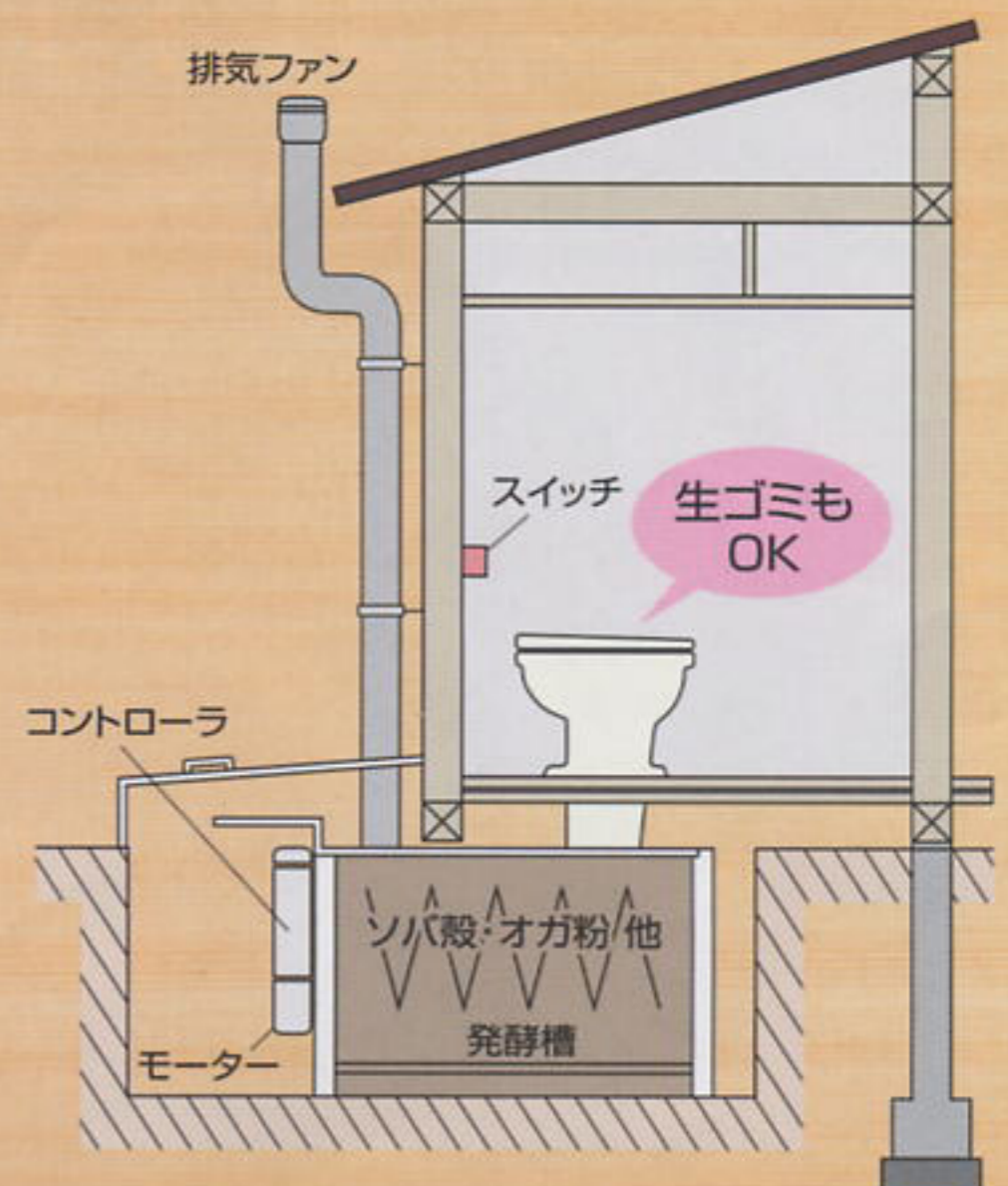
設置参考断面図
